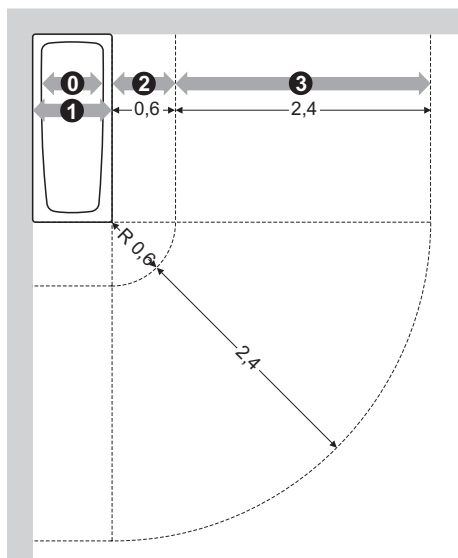
Bereichseinteilung bei Räumen mit Badewanne
